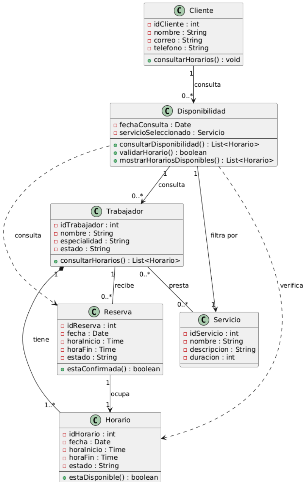
Diagrama de Clases - Visualizar Horarios de Trabajadores Disponibles
